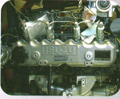
ISUZU C240
